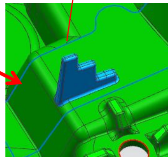
3指此形状交换入子形 状上有倒扣孔
